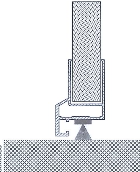
Schwellenlos mit Bürstendichtung
