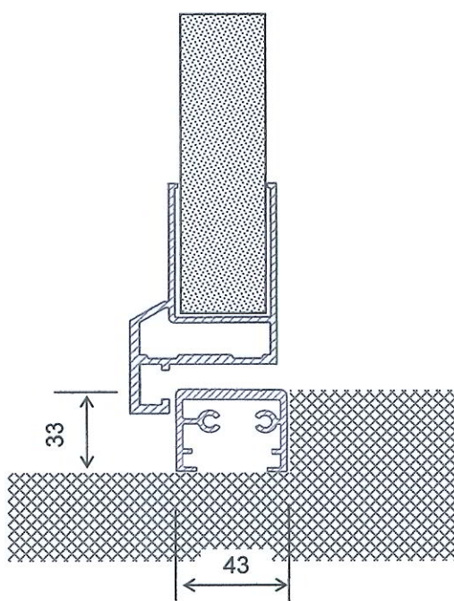
Bodenabschluss mit Schwelle
