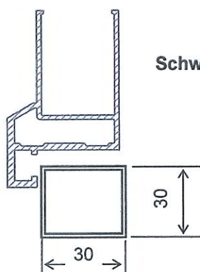
Schwellenprofile bei Blockrahmen
